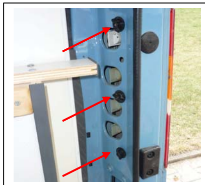
Rücklicht rechts. Kunststoff-Flügelschrauben lösen
