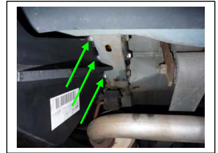
Montagepunkt AHK rechts. Scheiben als Distanz zwischen Rahmen und AHK
