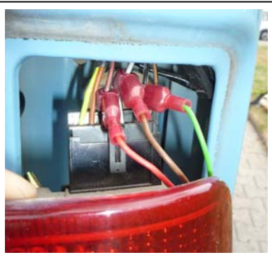
Anschluss E-Satz an Rücklicht rechts
