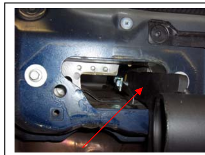
Tragarme in Chassis eingesteckt
