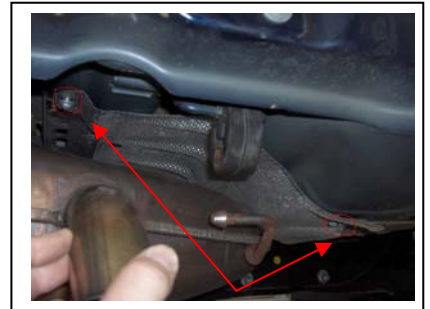
Nachschalldämpfer aushängen, Hitzeschild lösen
