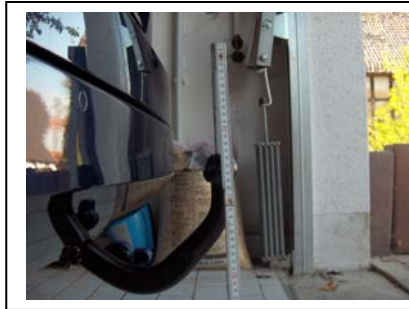
Kugelkopfabstand Fahrbahn – Kugel
