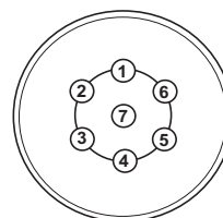
Laidų pajungimas 7 – pavažų lizdas
