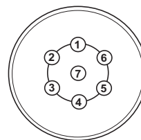
Kábelek bekötése a 7 pólusú dugaljba
