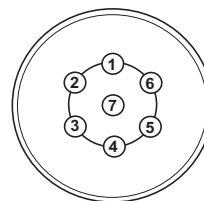
Подключение проводов в 7-полюсной розетке
