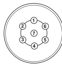
Johtojen liittyminen 7-napaiseen pistorasiaan
