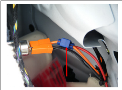
Dauerstrom Kabel mit Quetschverbinder an den Leiter der Kofferraumsteckdose
