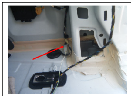
Verbindung für die PDC Abschaltung auf der rechten Seite
