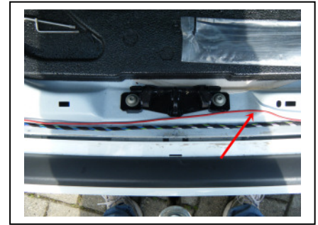
Dauerstrom Kabel Führung parallel zum Kabel der rechten Seite
