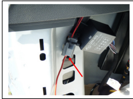
Dauerstrom Kabel mit 2,8 mm Flachverbinder in den Stecker
