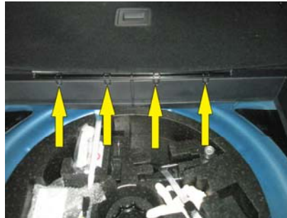
große Stauklappe durch lösen von 4 Torx- schrauben ausbauen
