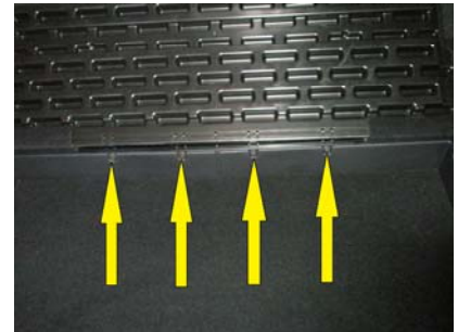
kleine Stauklappe durch lösen von 4 Torx- schrauben ausbauen
