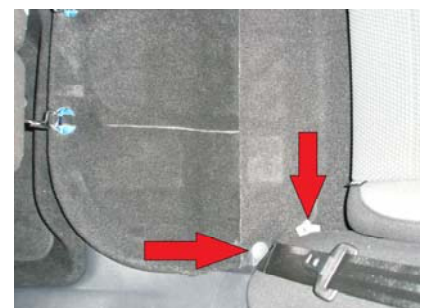
Sitzpolster im Fond hochklappen und die 2 Muttern entfernen
