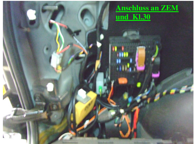
Einbaulage Anhängerkabelbaum und Steckdose
