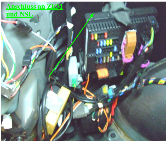
Einbaulage Kabelbaum und Steckdose
