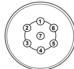
Connecteur des câbles le jack à 7 pôles
