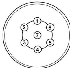
Johtojen liittyminen 7-nappaiseen pistorasiaan
