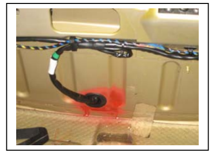
Kabelbaum durch Heck- blech durchgeführt
