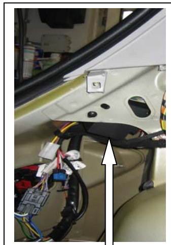
verbautes Überwachungs- modul (hinter linker Koffer- raumverkleidung und teil- weise hinter C-Säule)
