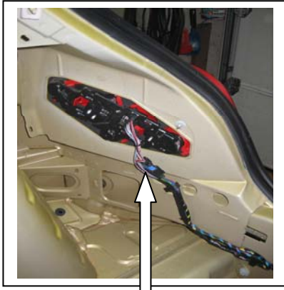
montierter Kabelbaum an der rechten Rückleuchte
