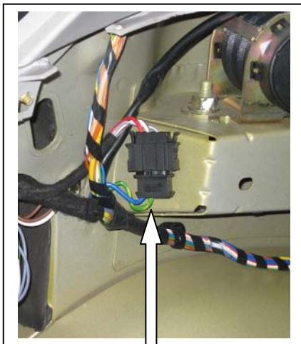
Spannungsversorgung des Überwachungsmoduls (Anschluss über den mitge- lieferten Flachstecker nach Umbau)
