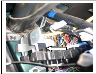
Blinkrelais
