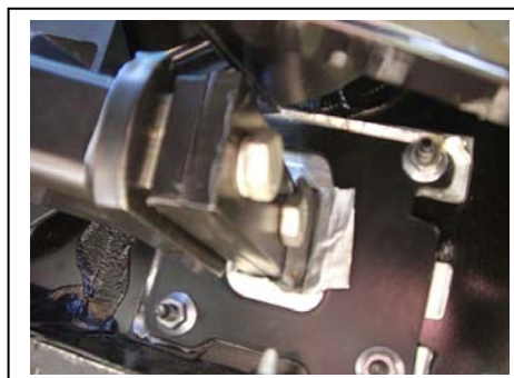
Verschraubung AHK-Träger mit Befestigungseisen rechts (17-er und 19-er)
