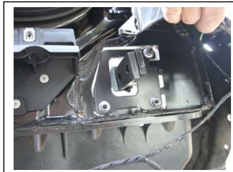
Befestigungseisen im rechten Längsträger mit eingeschnittener Abdeckung und Verschraubung
