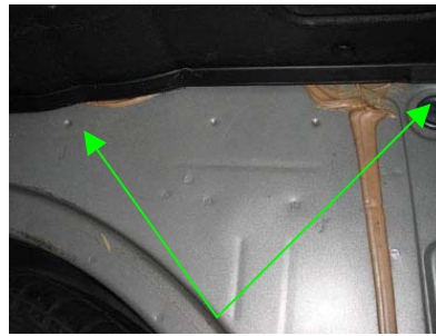
Montagepunkte rechts
